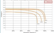
不同環境溫度下LYP鋰電池的放電特性曲線 LFP battery's discharge curve under different temperatures
